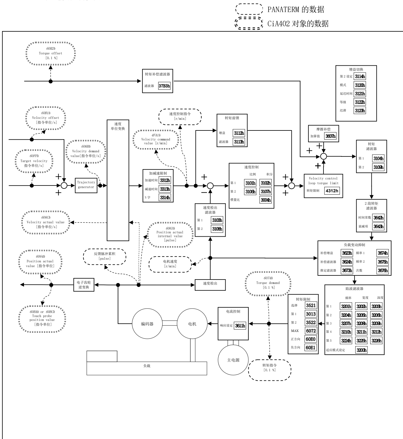
速度控制框图
