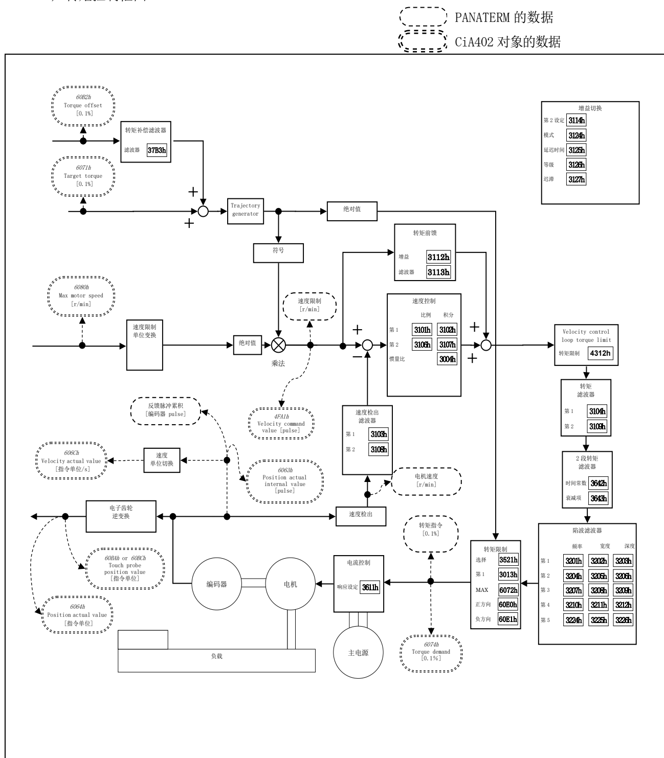
转矩控制框图
