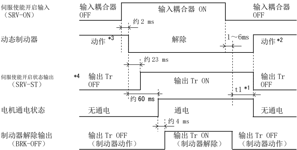
9-2-2 电机停止（伺服锁定）时的伺服使能开启/关闭动作时序图 （通常动作时使电机停止后再进行伺服使能开启/关闭动作。）
