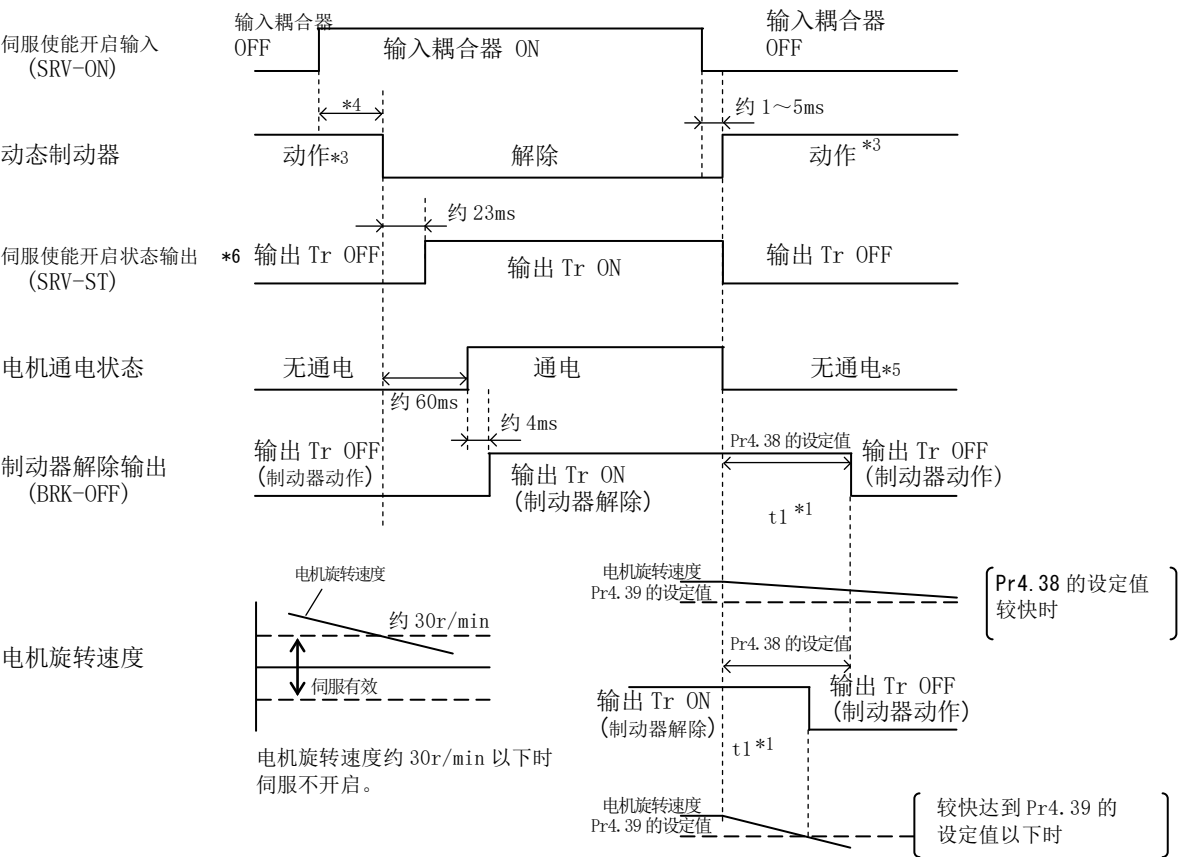
9-2-3 电机旋转时的伺服使能开启/关闭动作时序图 (紧急停止或者跳闸时的时序图，不可重复使用。)
