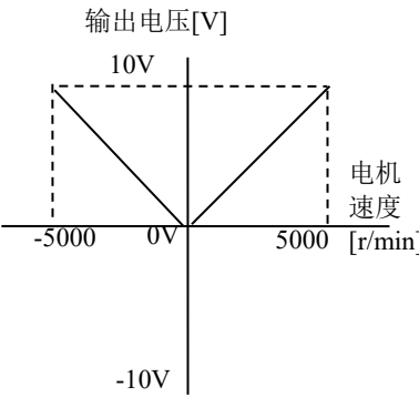
Pr4.21=1 绝对值数据输出 (输出范围 0~10 V)
