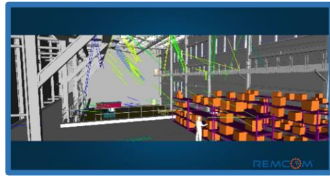
■ 工厂/仓储环境中的 5G 无线网络规划
