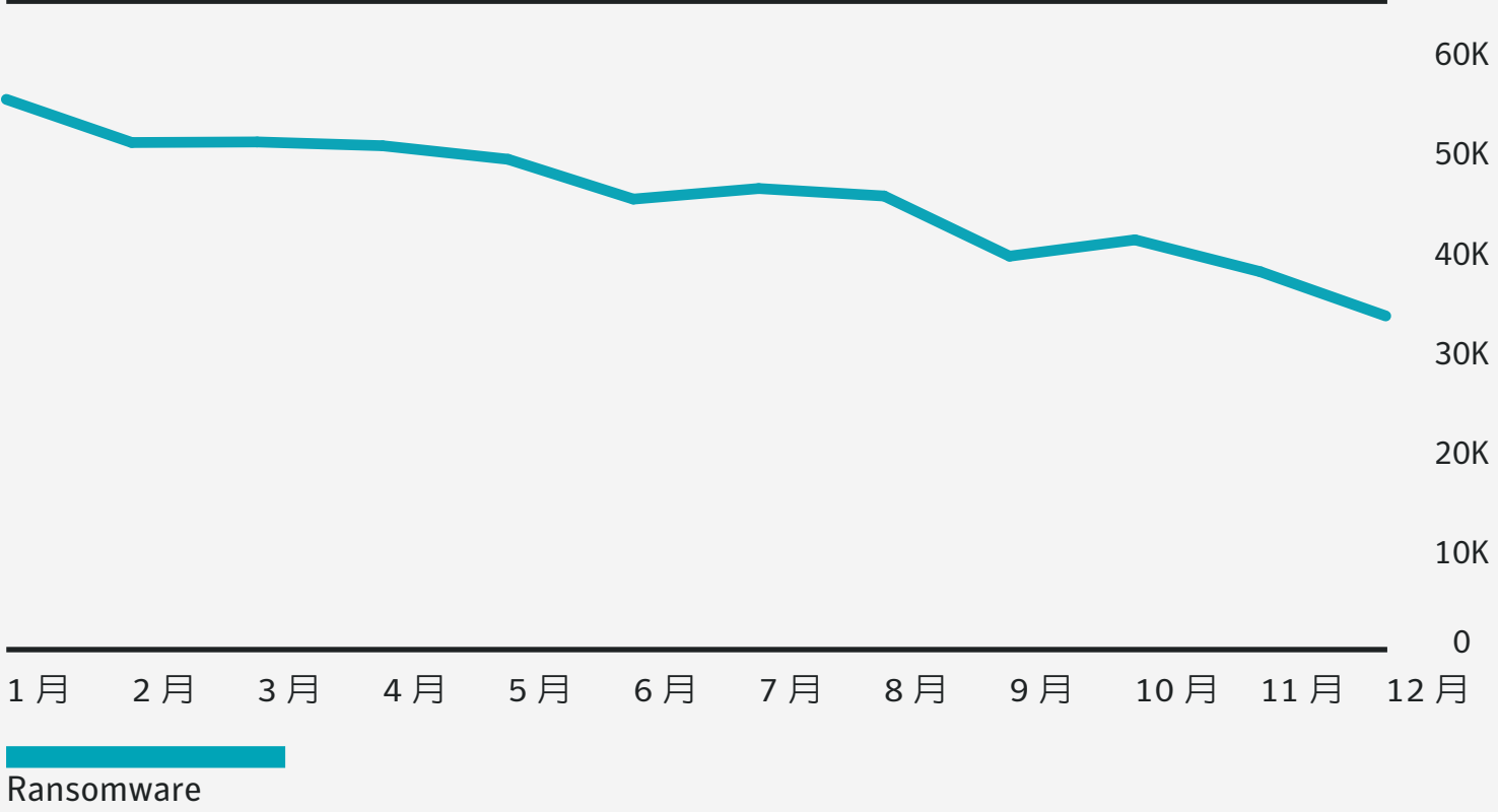
勒索軟體總數 (月)
