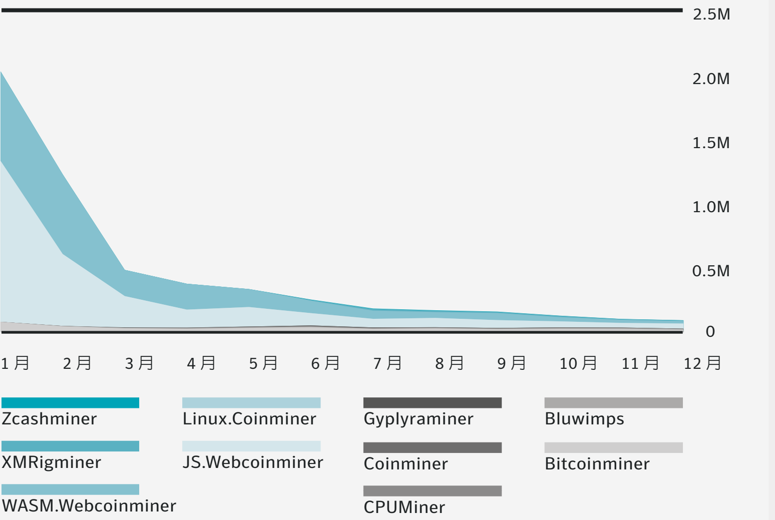
熱門加密貨幣挖礦程式 (月)
