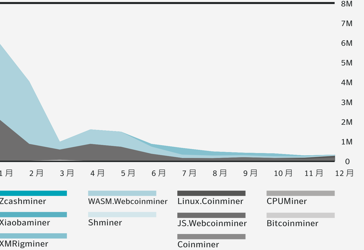
惡意程式：熱門加密貨幣挖礦程式變種 (月)
