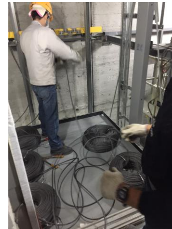
日期： 12/29 施作內容： B棟電梯纜線施作
