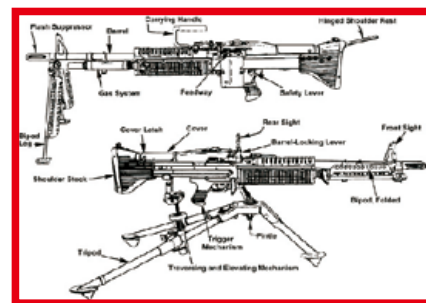
M60的線圖與M122腳架組合示意圖。(By www.gun.com)
