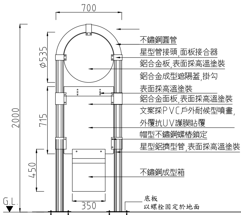
立面圖
