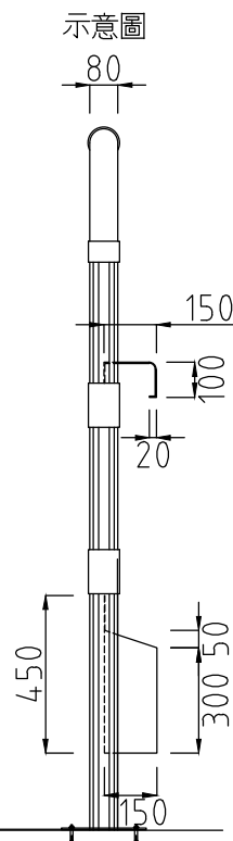
側立面圖
