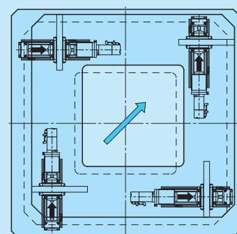
XY运动
