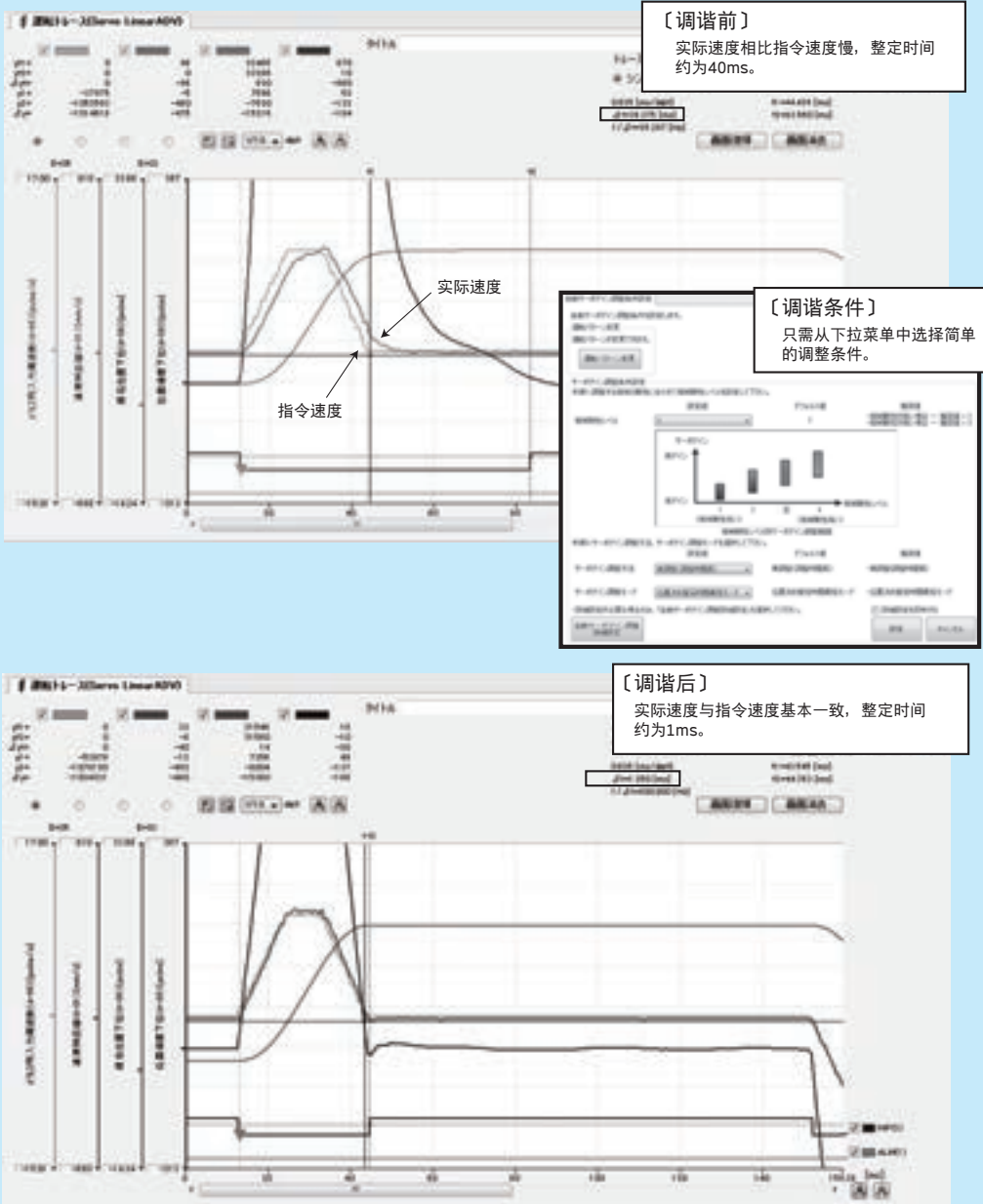
图2 自动调谐
