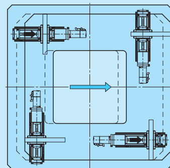
X运动
