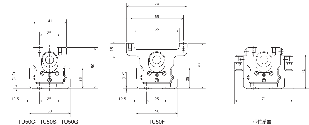
A-A 断面尺寸
