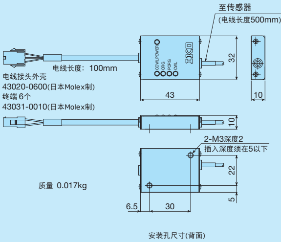
图1 传感器放大器的外形尺寸
