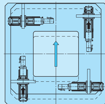
Y运动
