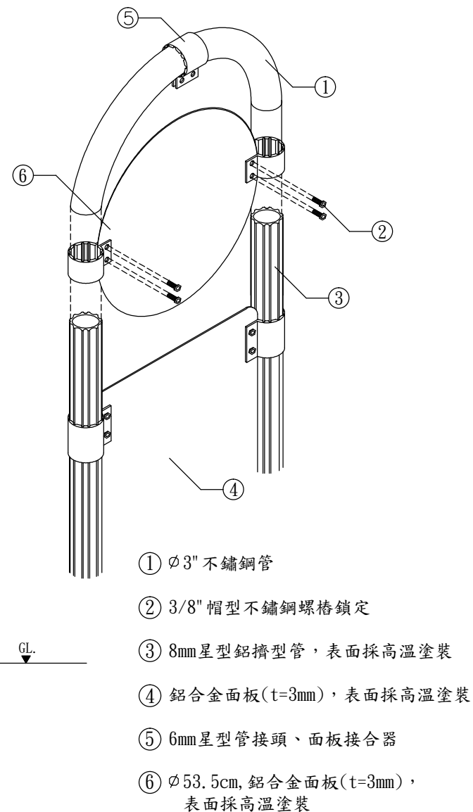
面板接合詳圖
