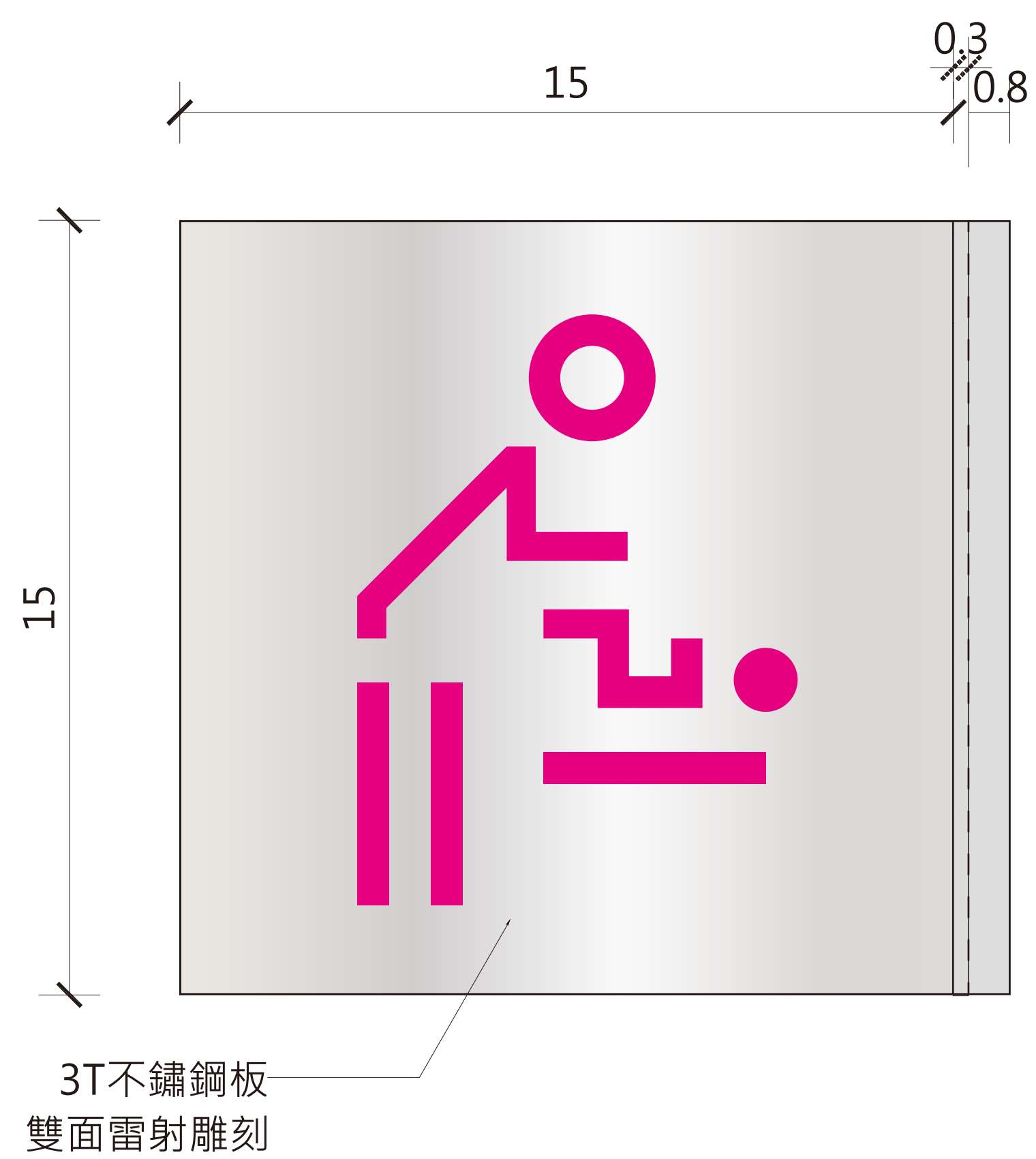
4 親子廁所指標平面圖x1 Scale: 1/3(A3) Units:cm 1/1.5(A1)
