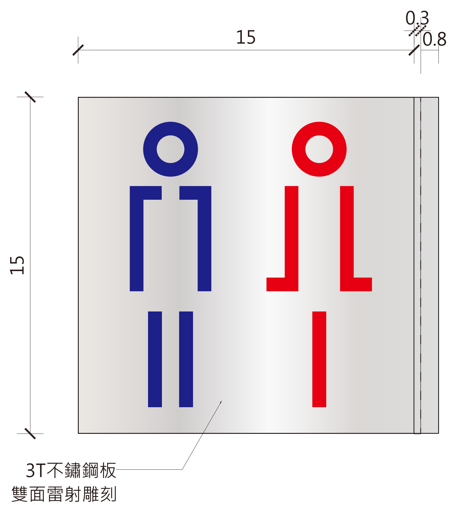
7 廁所主入口指標平面圖x1 Scale: 1/3(A3) Units:cm 1/1.5(A1)
