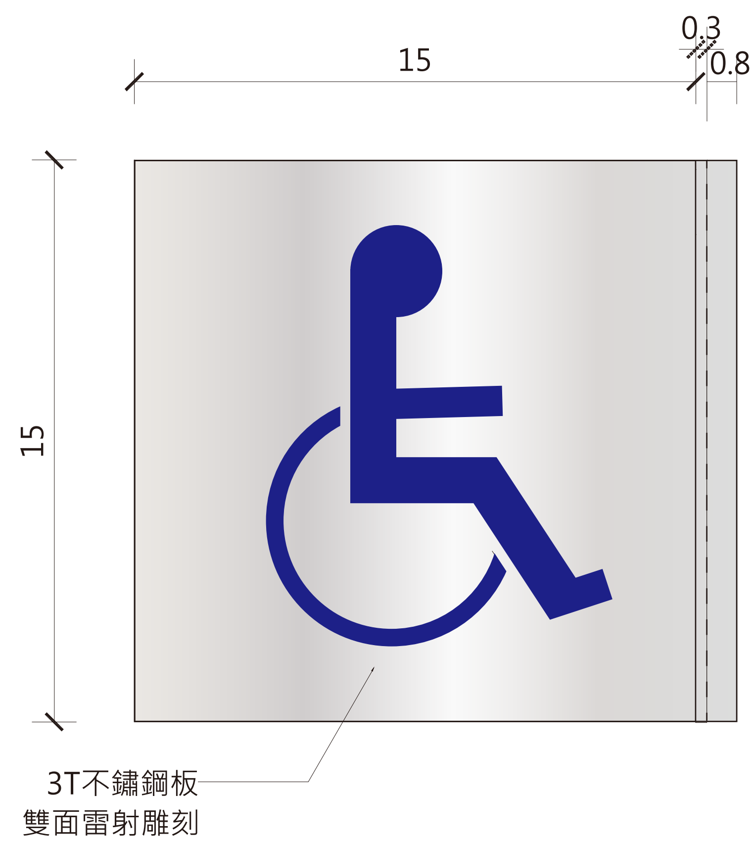
3 無障礙廁所指標平面圖x1 Scale: 1/3(A3) Units:cm 1/1.5(A1)
