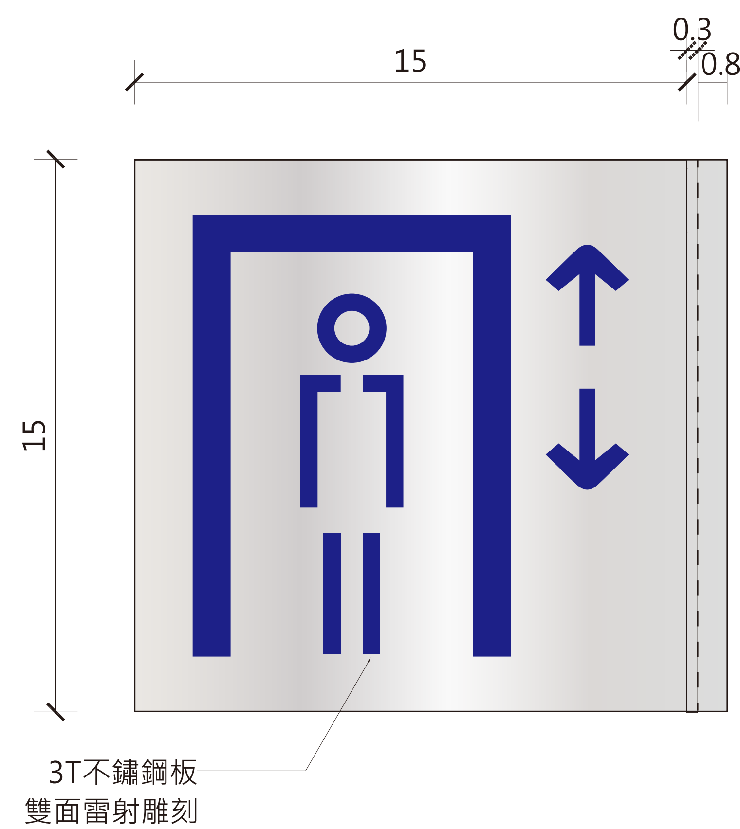
8 電梯指標平面圖x1 Scale: 1/3(A3) Units:cm 1/1.5(A1)
