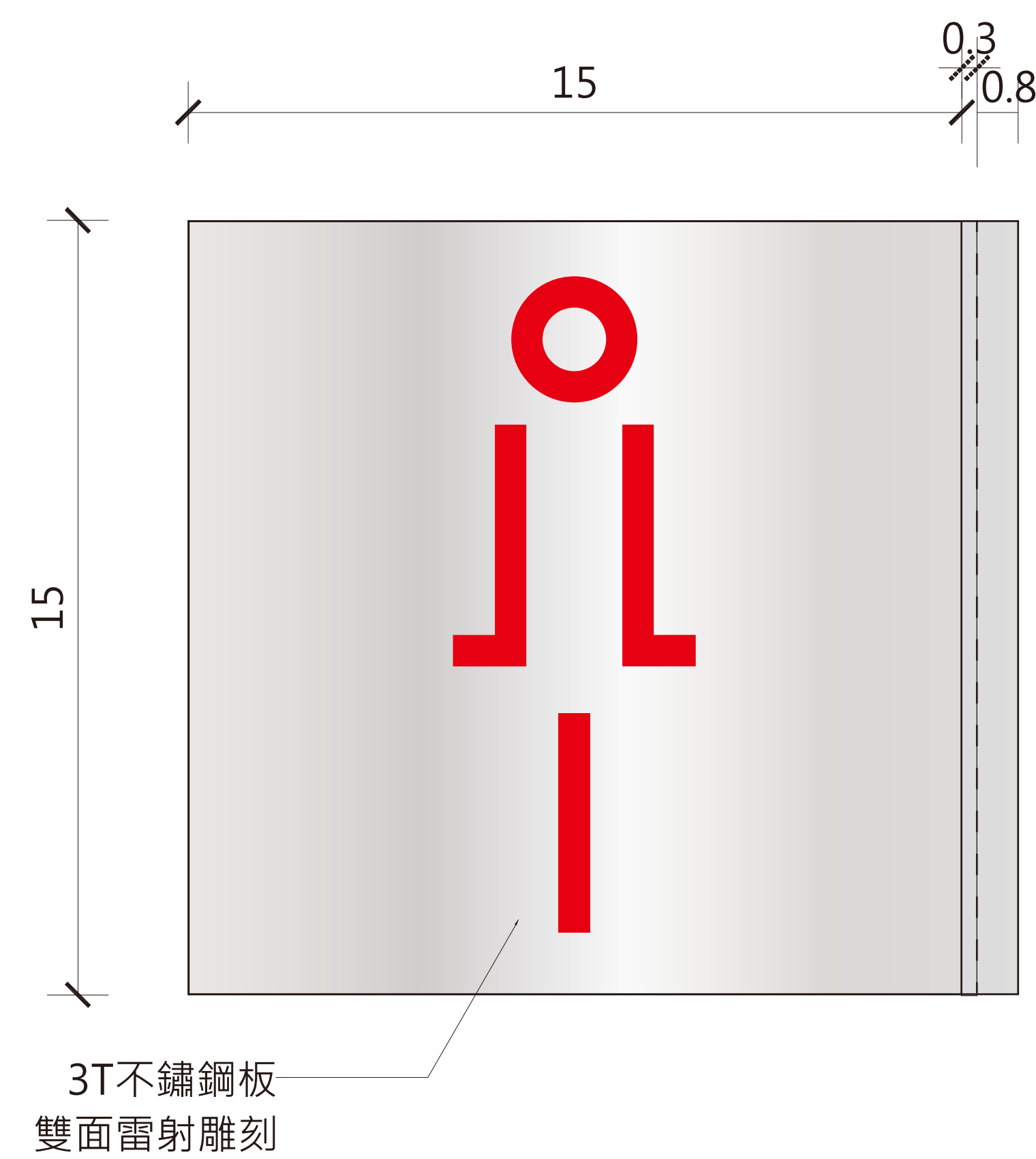
5 女生廁所指標平面圖x1 Scale: 1/3(A3) Units:cm 1/1.5(A1)
