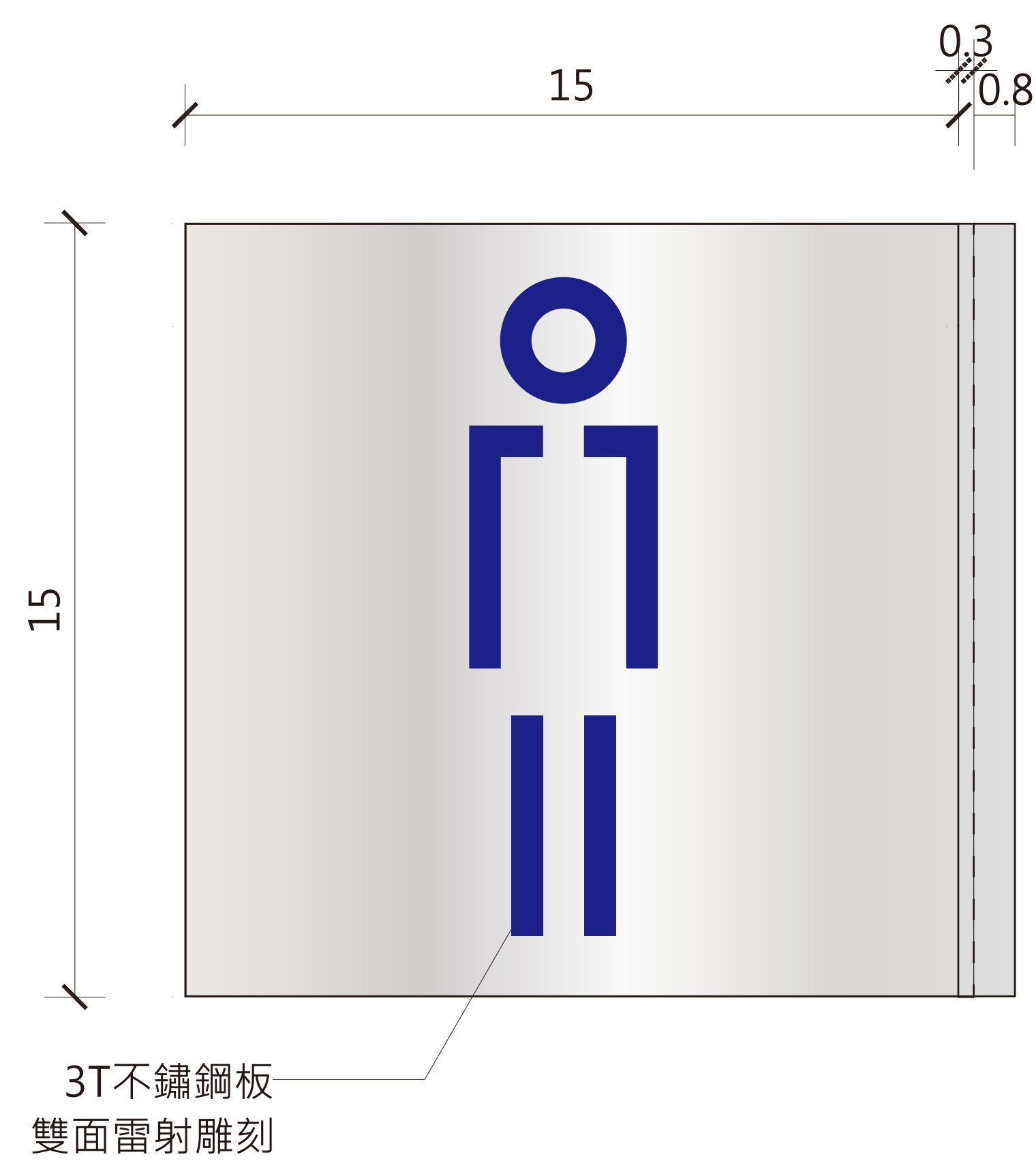
6 男生廁所指標平面圖x1 Scale: 1/3(A3) Units:cm 1/1.5(A1)
