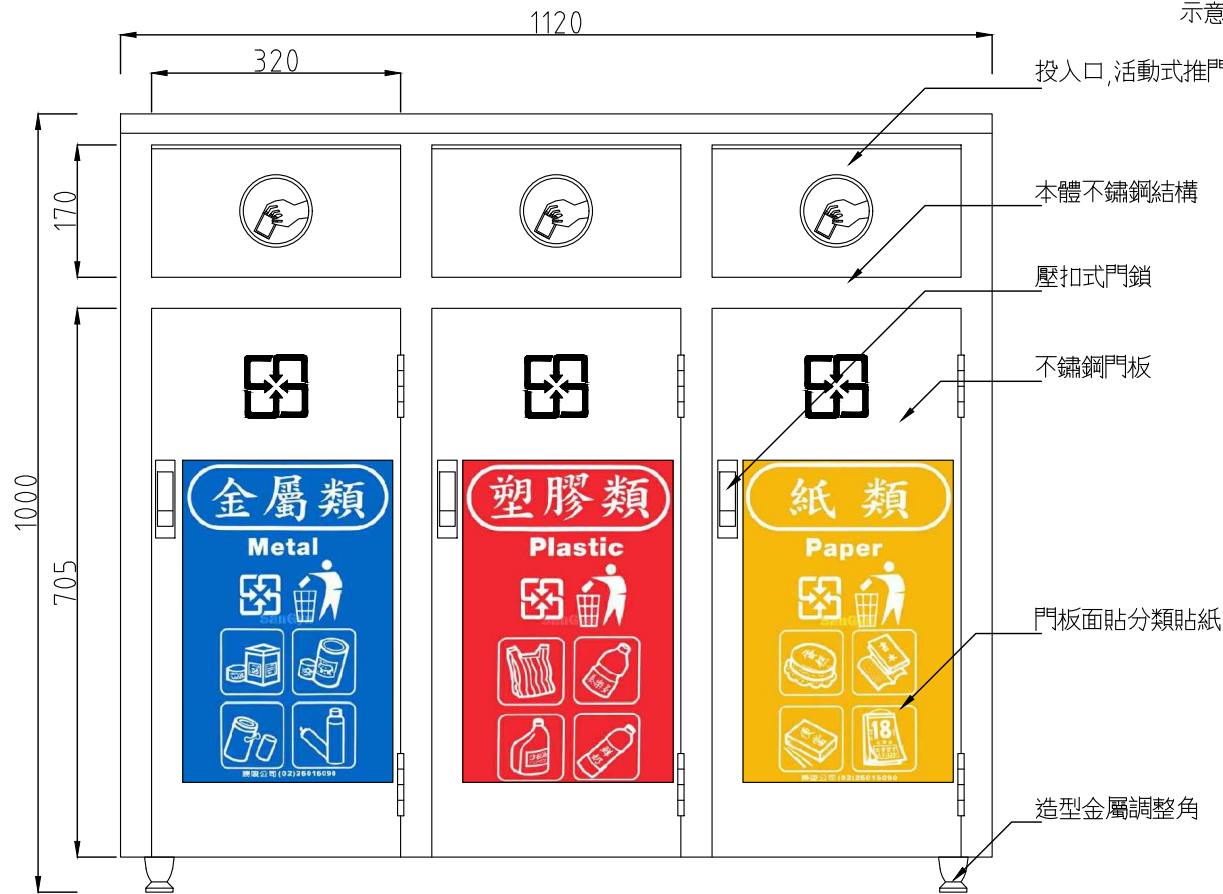
立面圖
