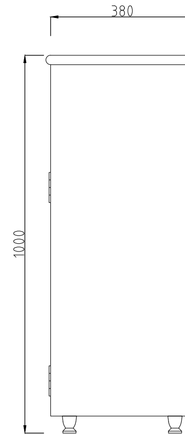
側立面圖
