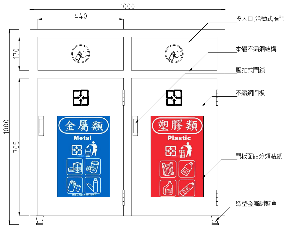
立面圖
