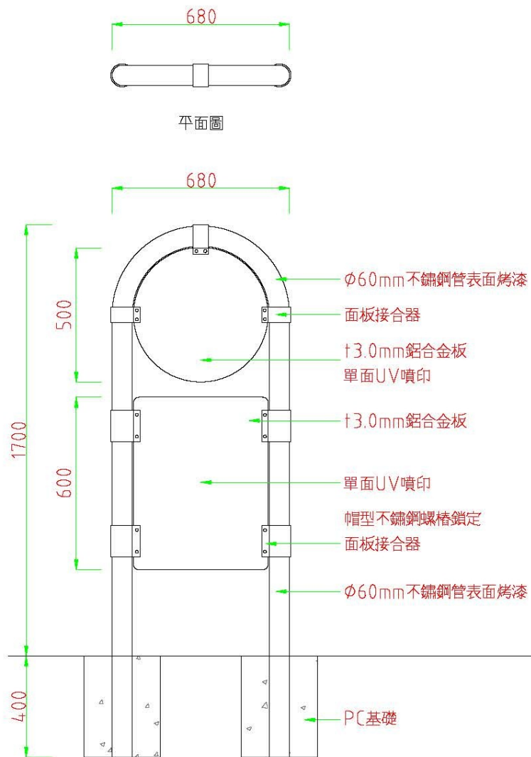
立面圖
