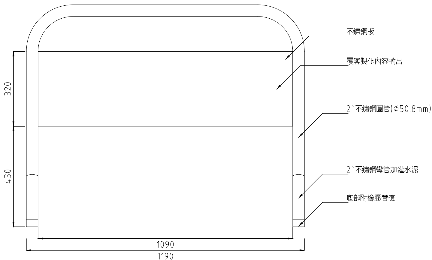
立面圖
