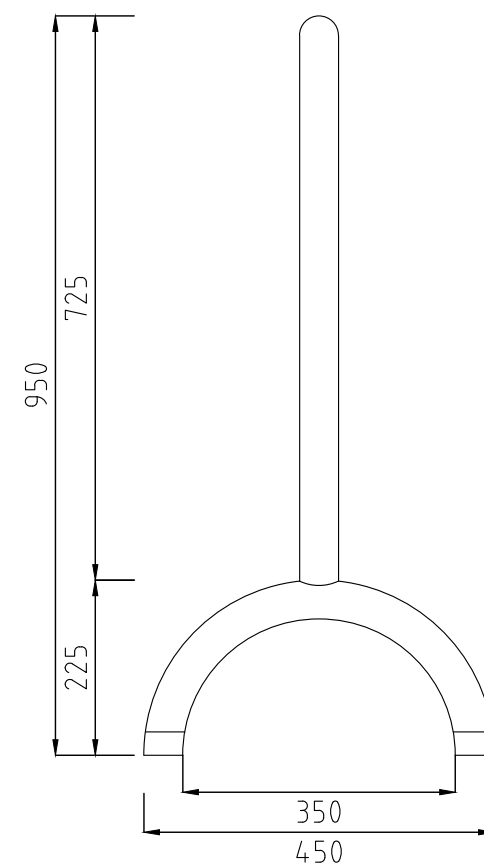
側立面圖
