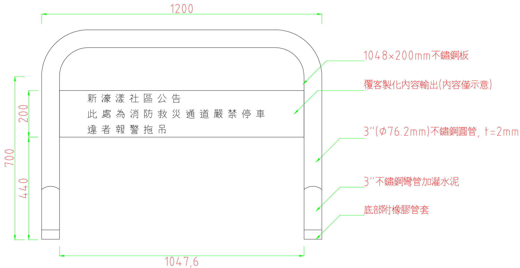
立面圖
