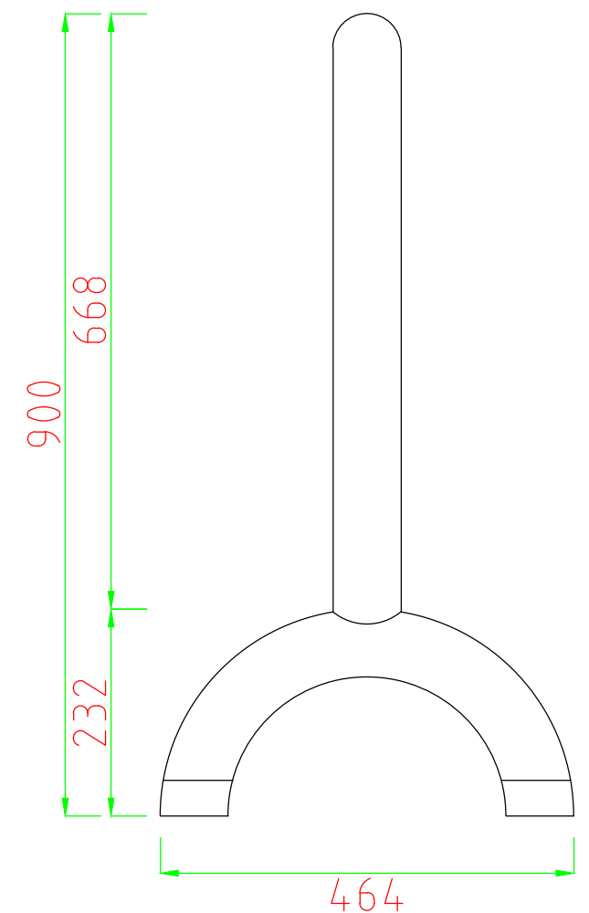
側立面圖
