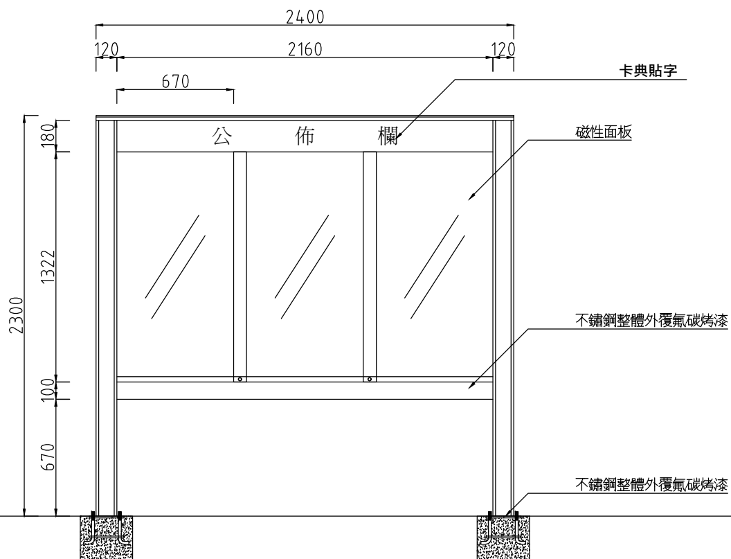
立面圖
