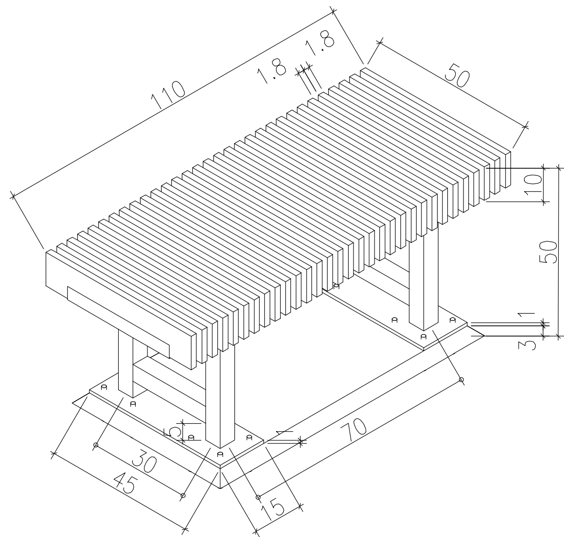
3 座椅詳圖 單位:公分 A5-03 scale:A1 1/10 A3 1/20
