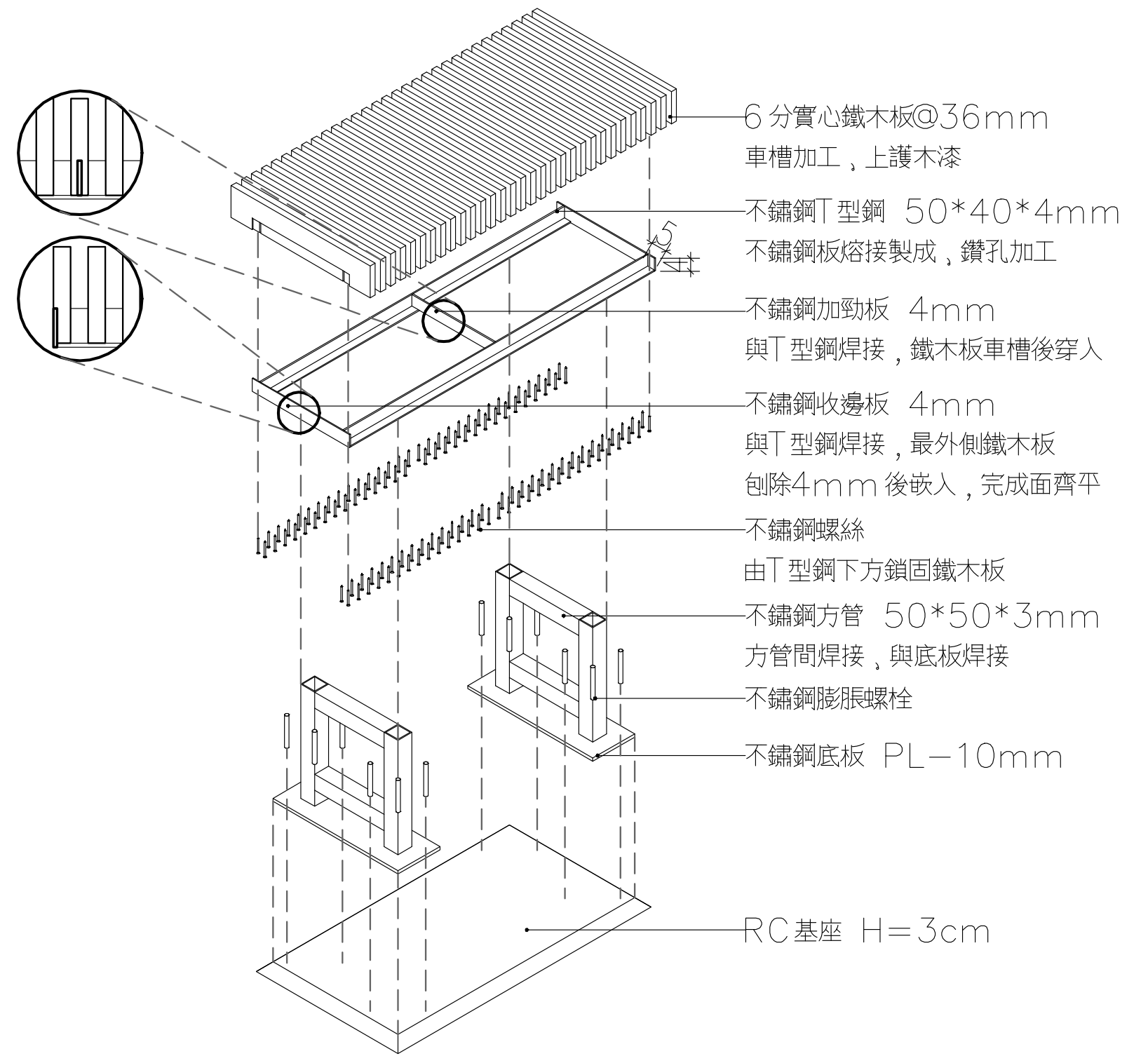
3 座椅構成爆炸圖 A5-03 scale:A1 1/15 A3 1/30
