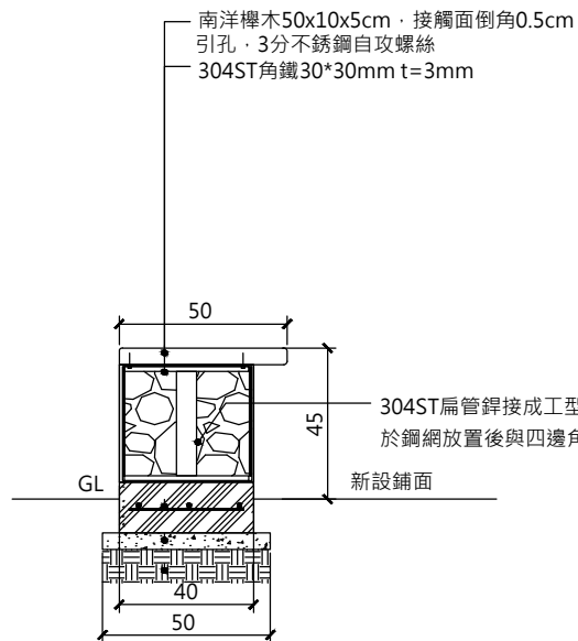
1 休憩座椅-A大樣圖 A3 : 1/20 A1 : 1/10 U=cm
