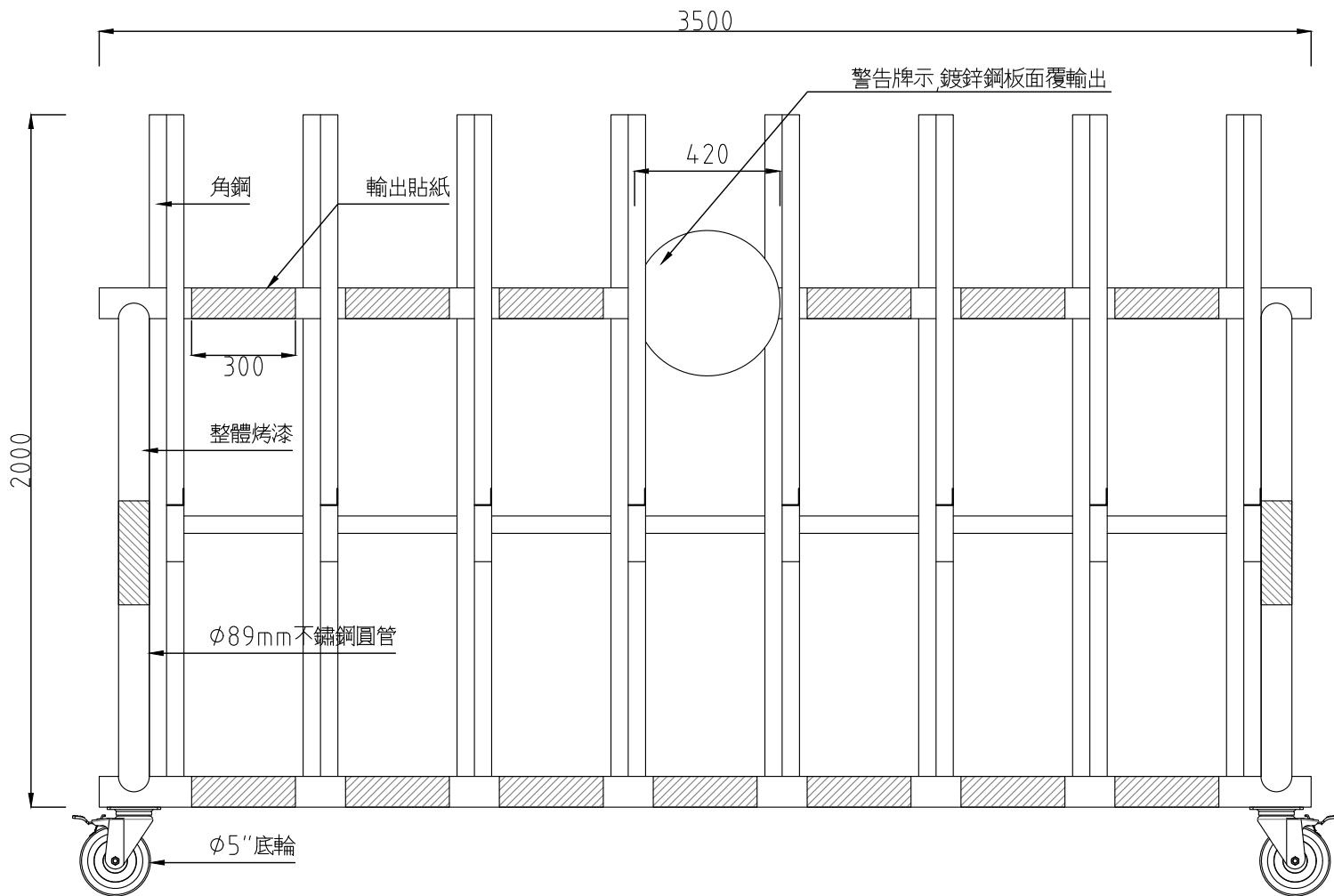
立面圖
