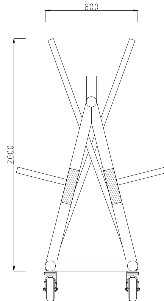
側立面圖
