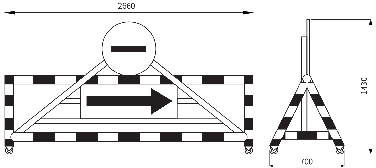
大型不鏽鋼阻隔拒馬 示意圖
