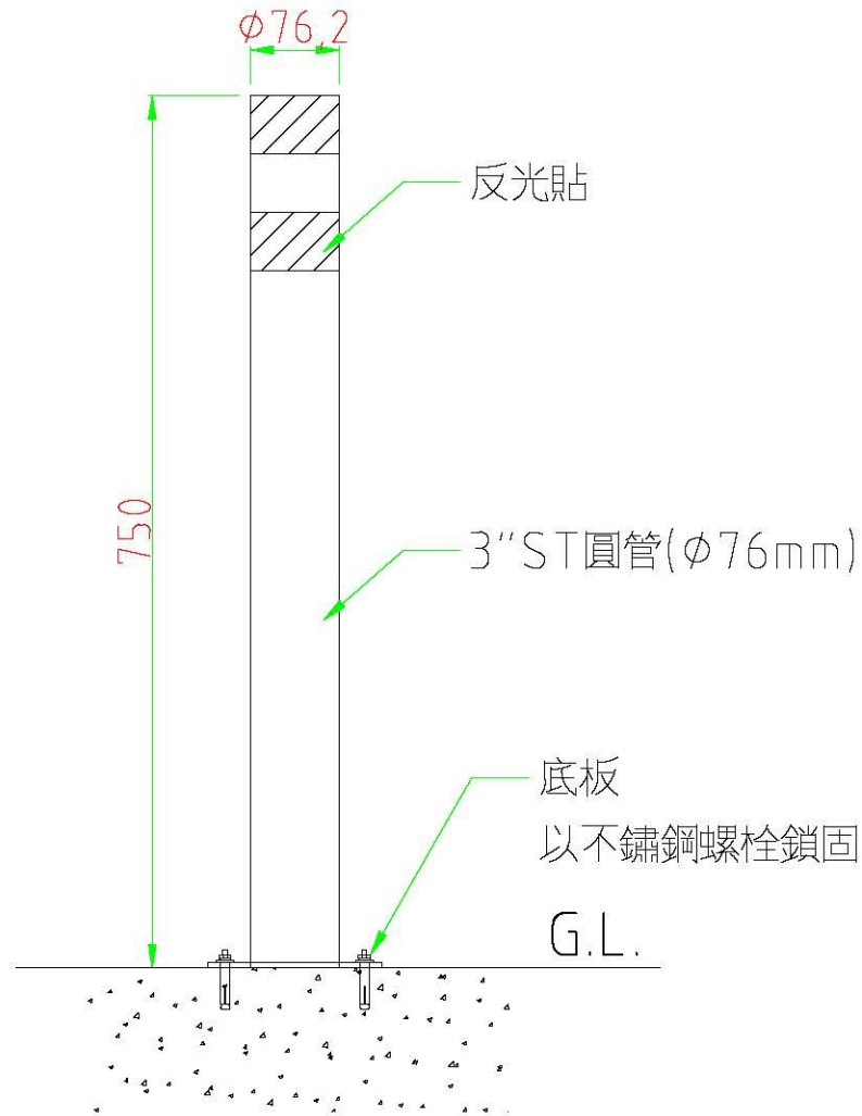
示意圖 立柱型
