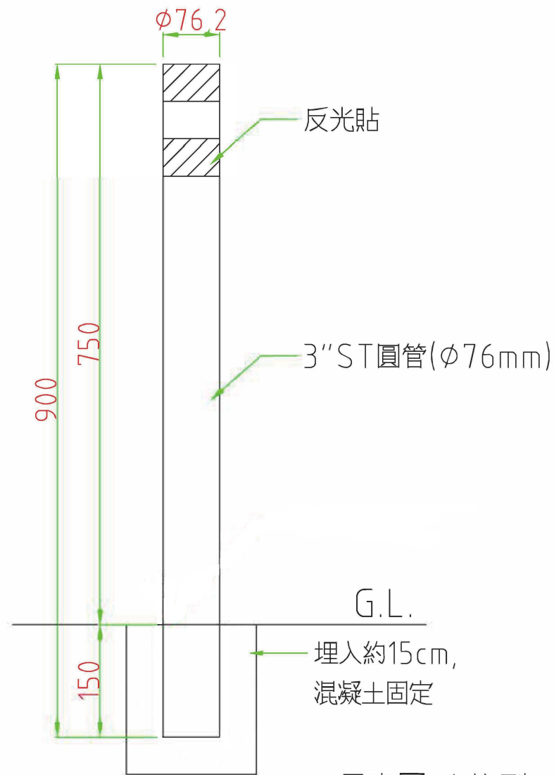
示意圖 立柱型
