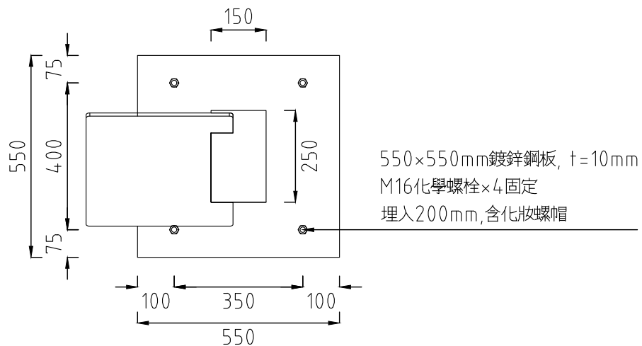
平面圖
