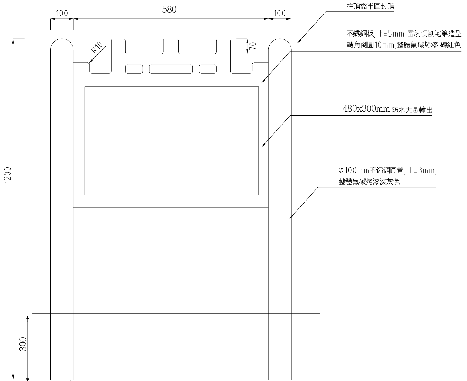
立面圖
