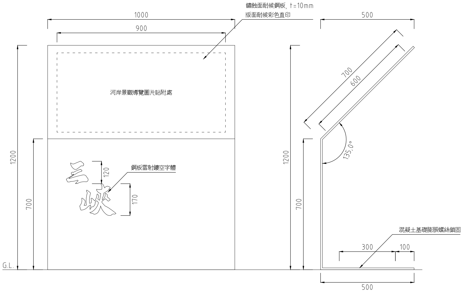
立面圖
