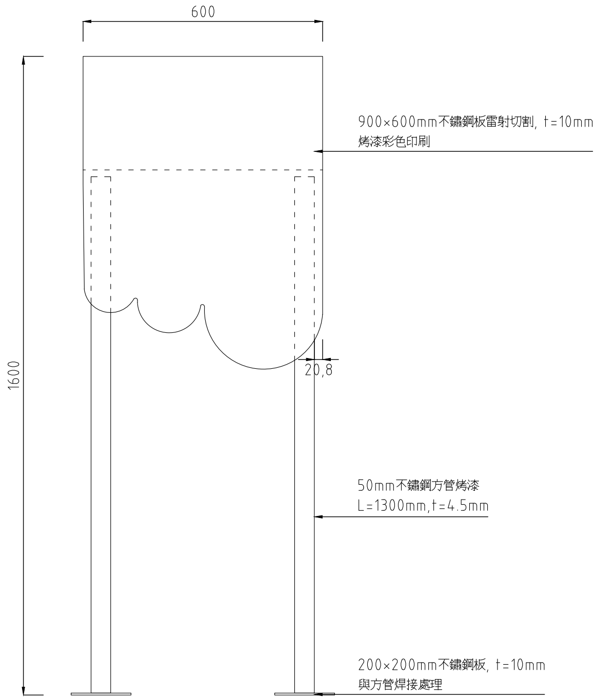
立面圖
