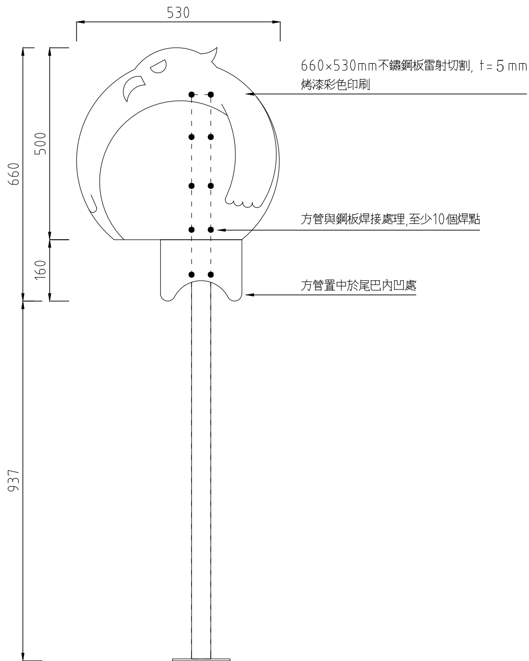
立面圖
