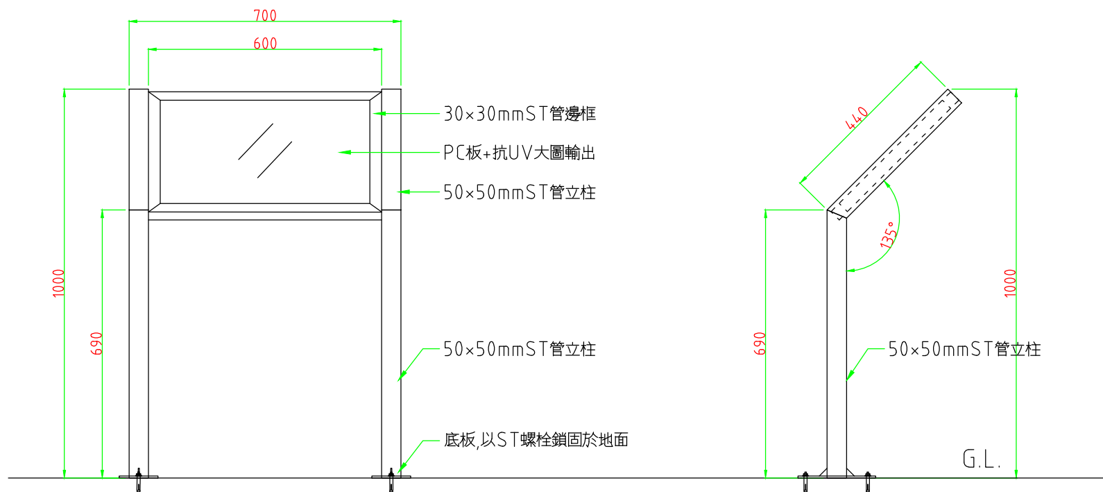
正立面圖
