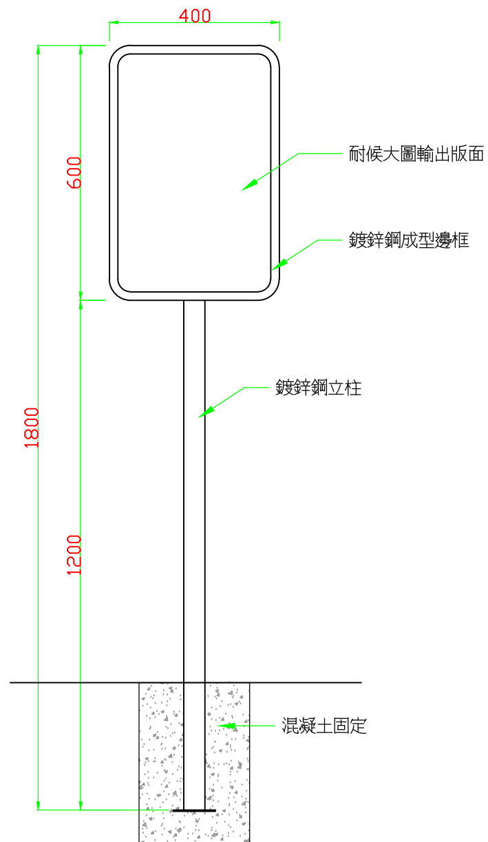
正視圖
