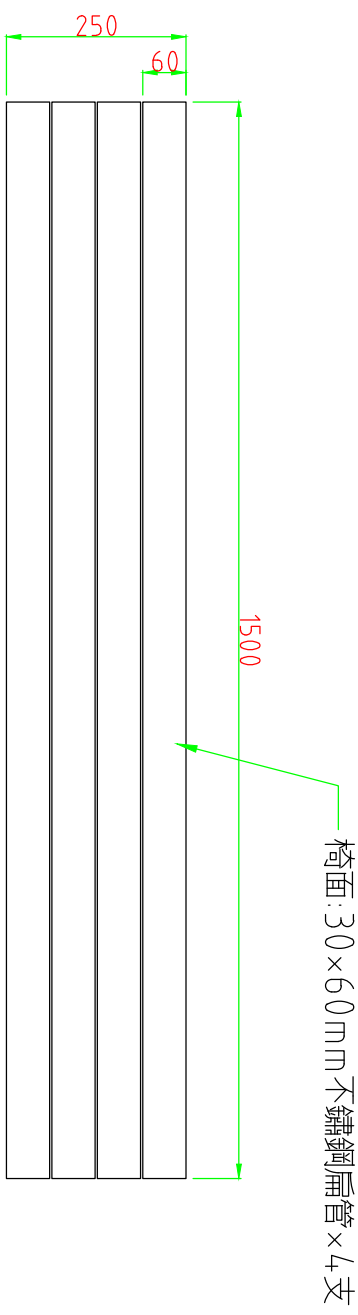
平面圖
