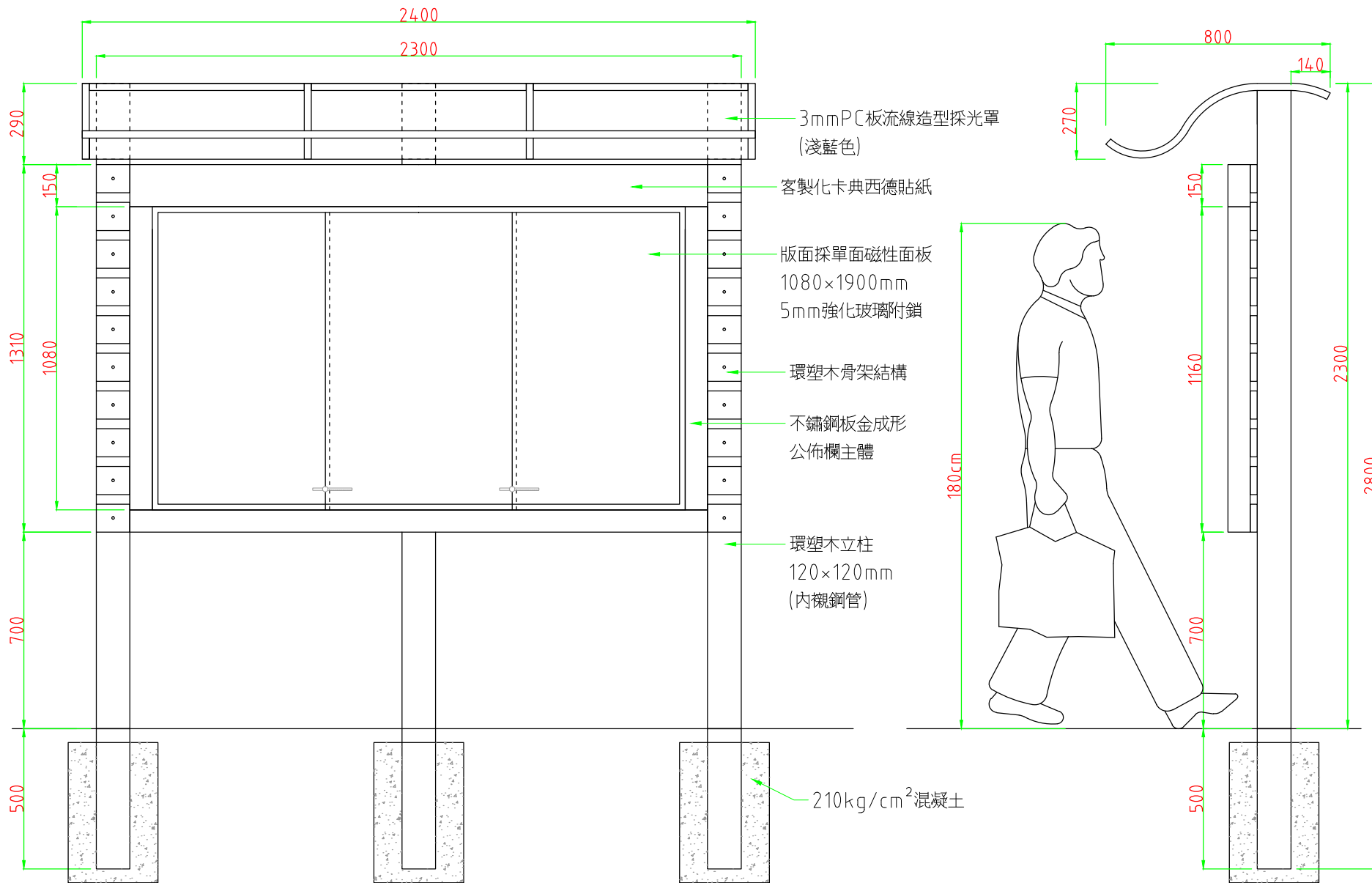
正視圖
