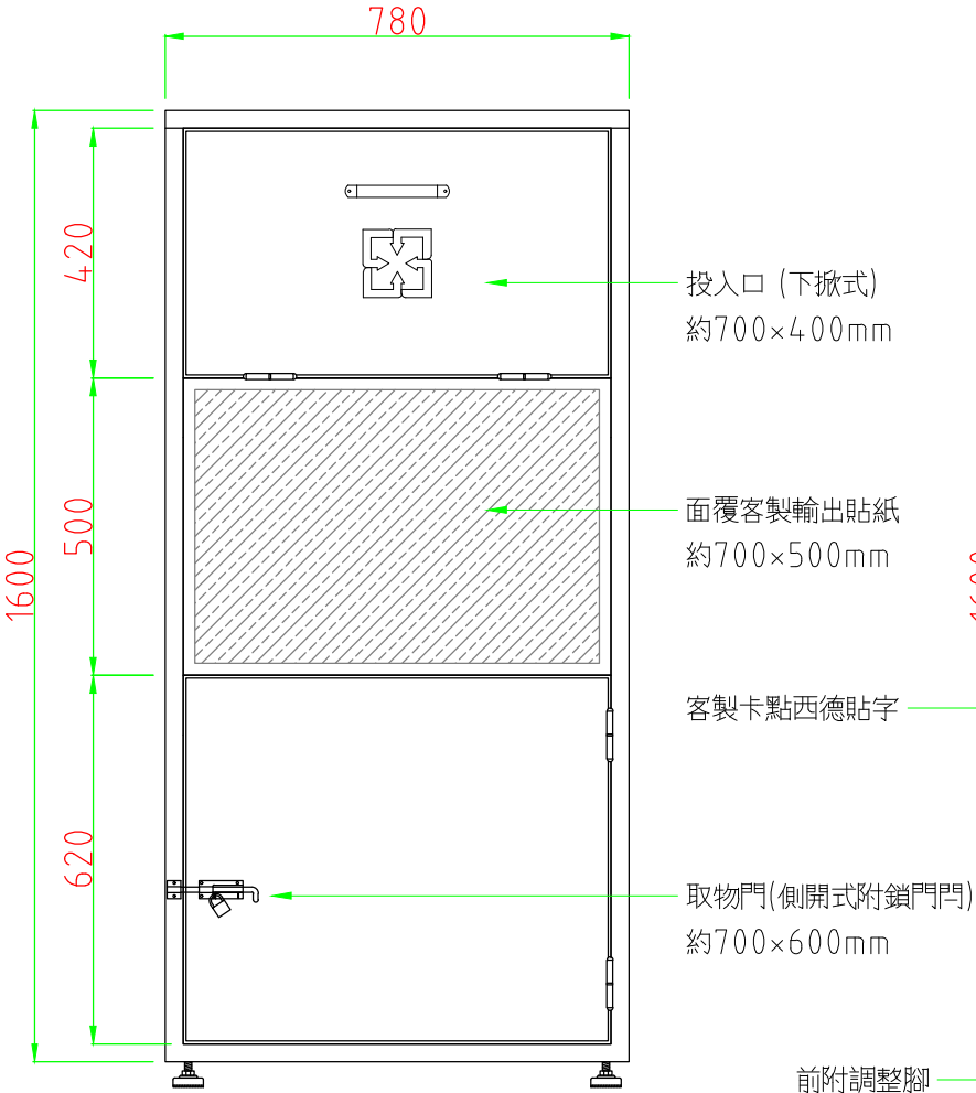
正立面圖
