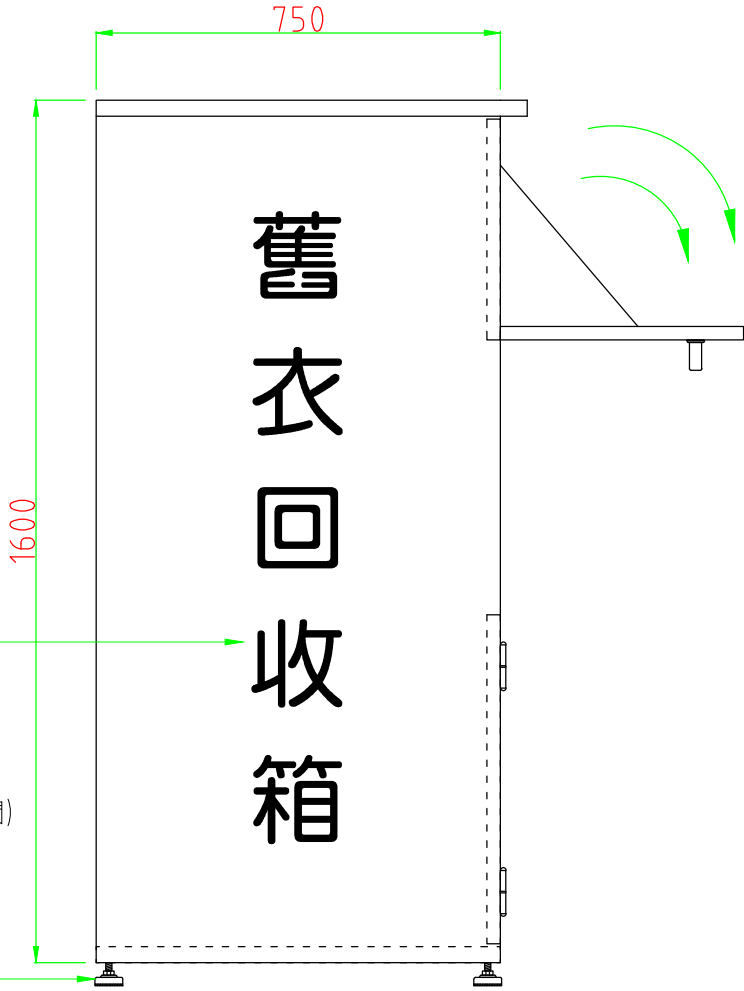
側立面圖
