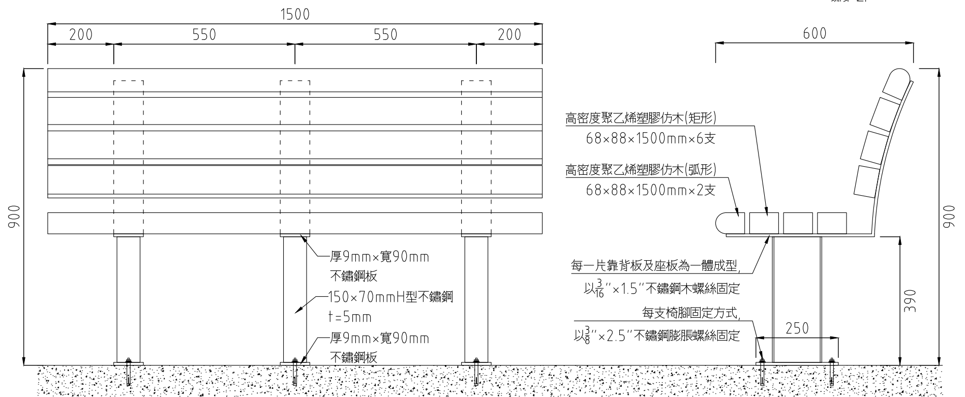
立面圖
