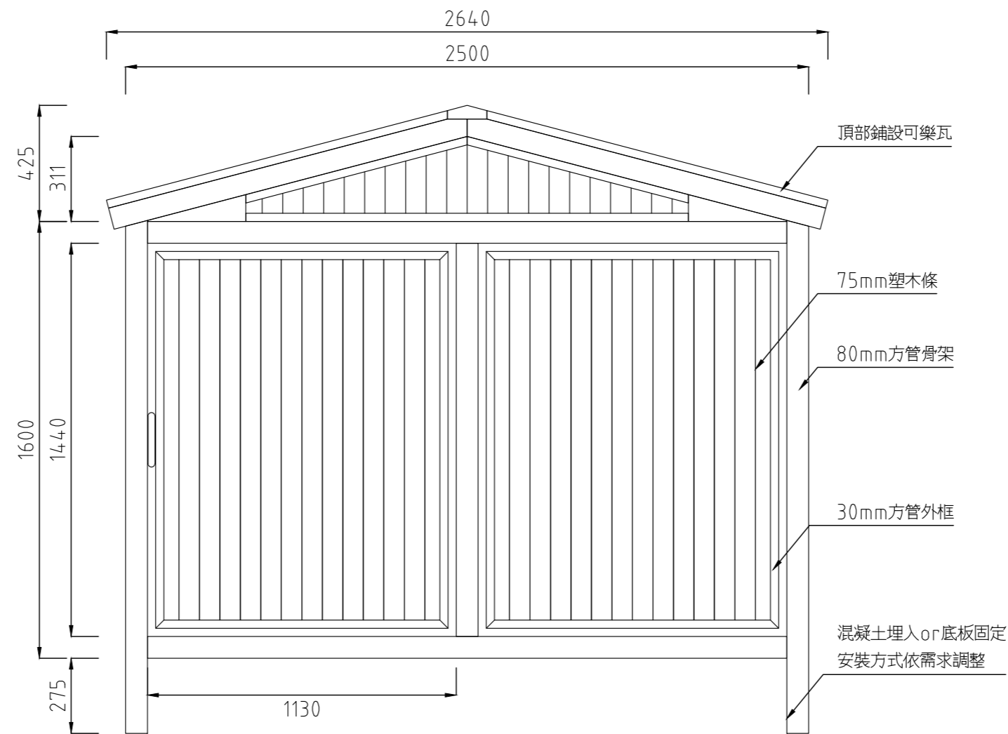
立面圖
