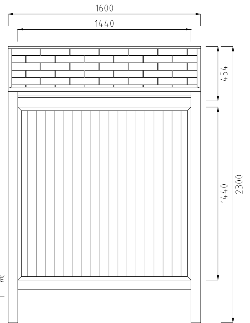
側立面圖
