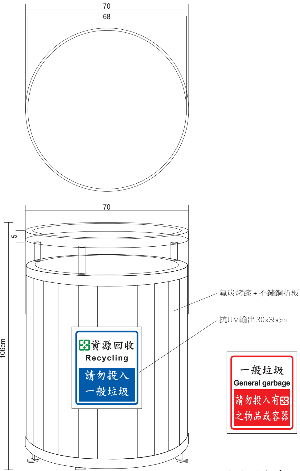
全部尺寸(±2%)mm
