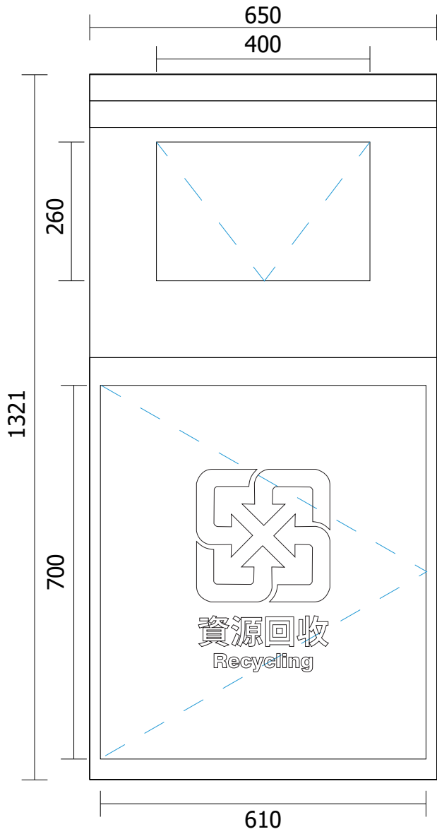
正視圖
