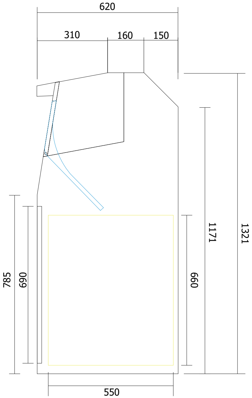
側視圖(關閉)
