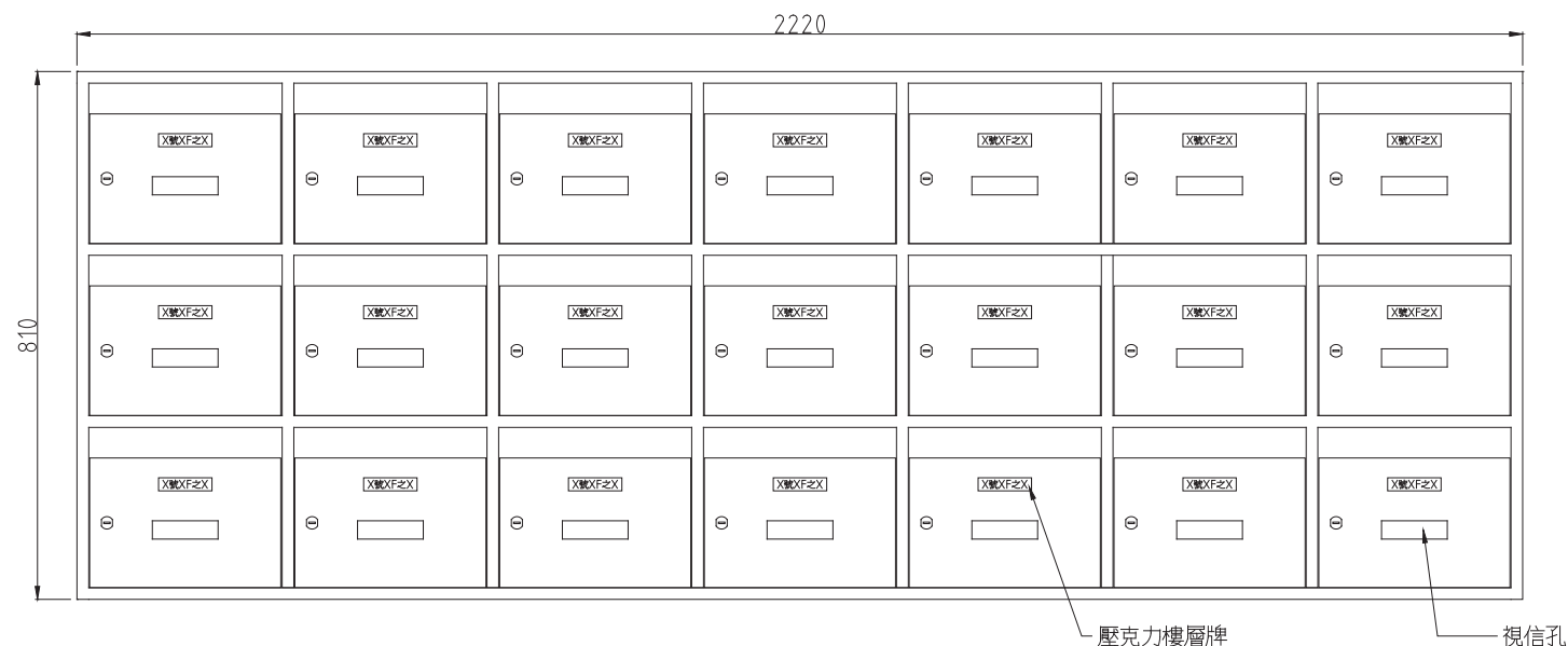
連體信箱 示意圖 (共21戶) 尺寸:L2220×H810×D100mm
