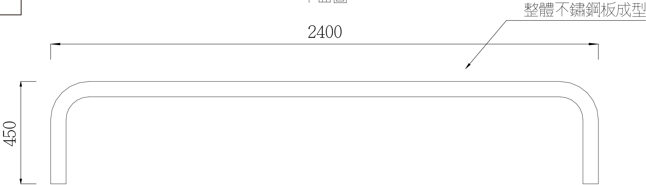
平面圖
