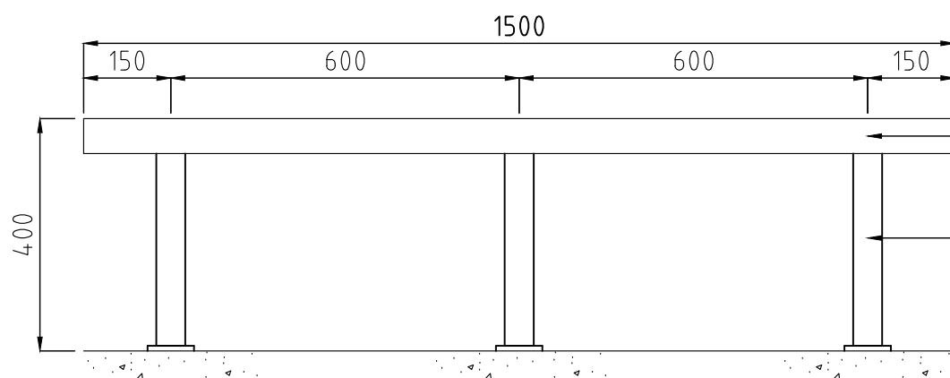
背立面圖
