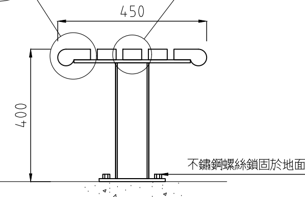
側立面圖
