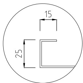
門板平剖詳圖
