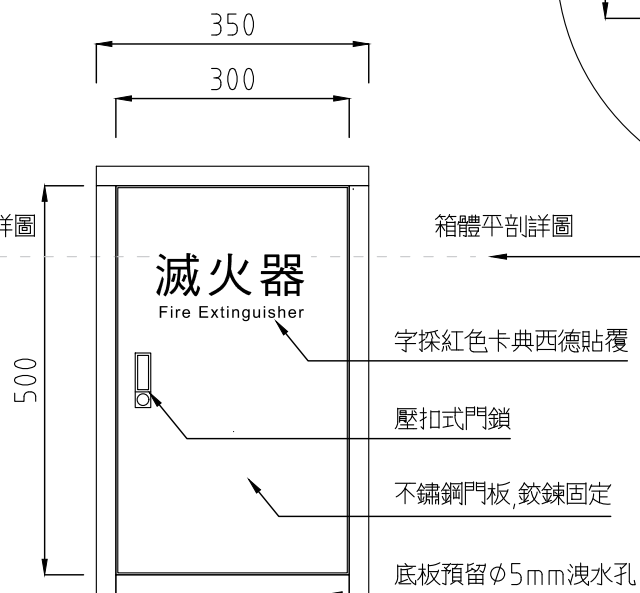
立面圖
