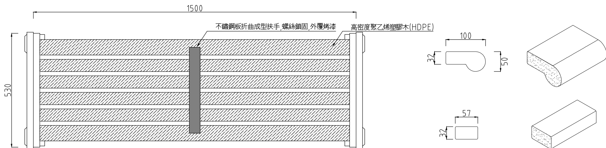
平面圖
