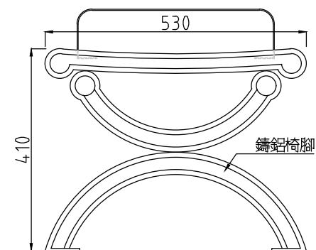
側立面圖
