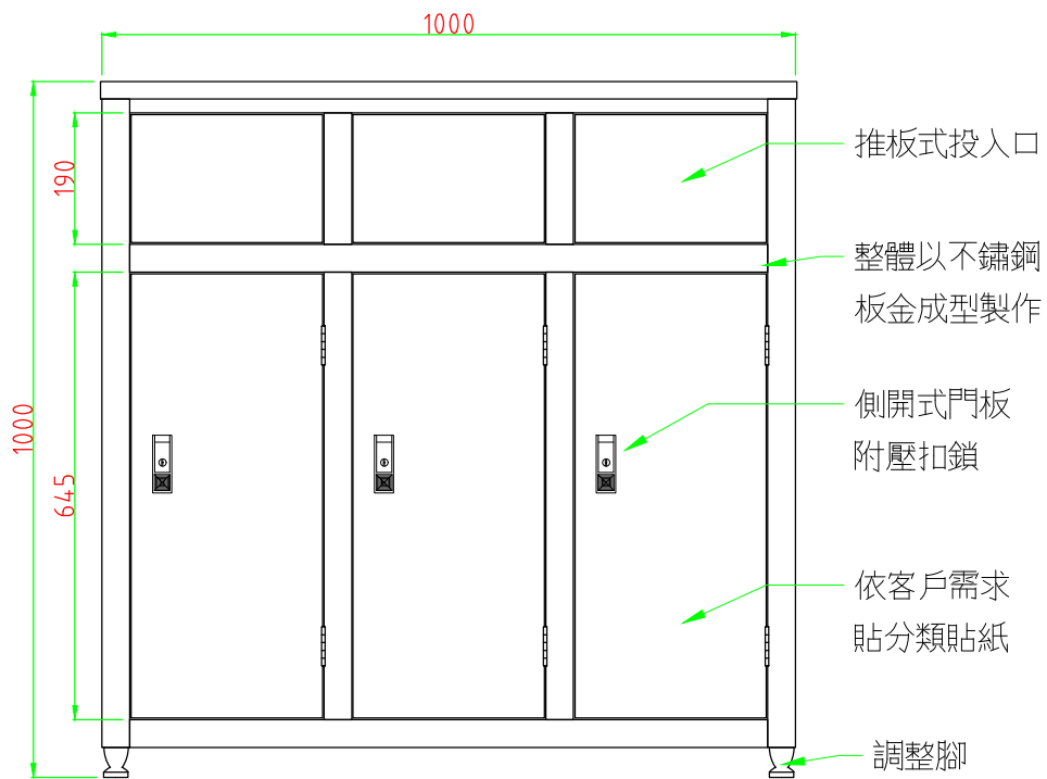
正視圖
