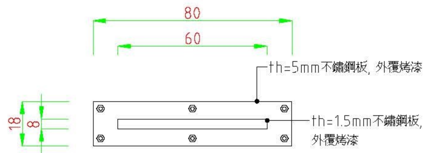
公園導覽牌上視圖
