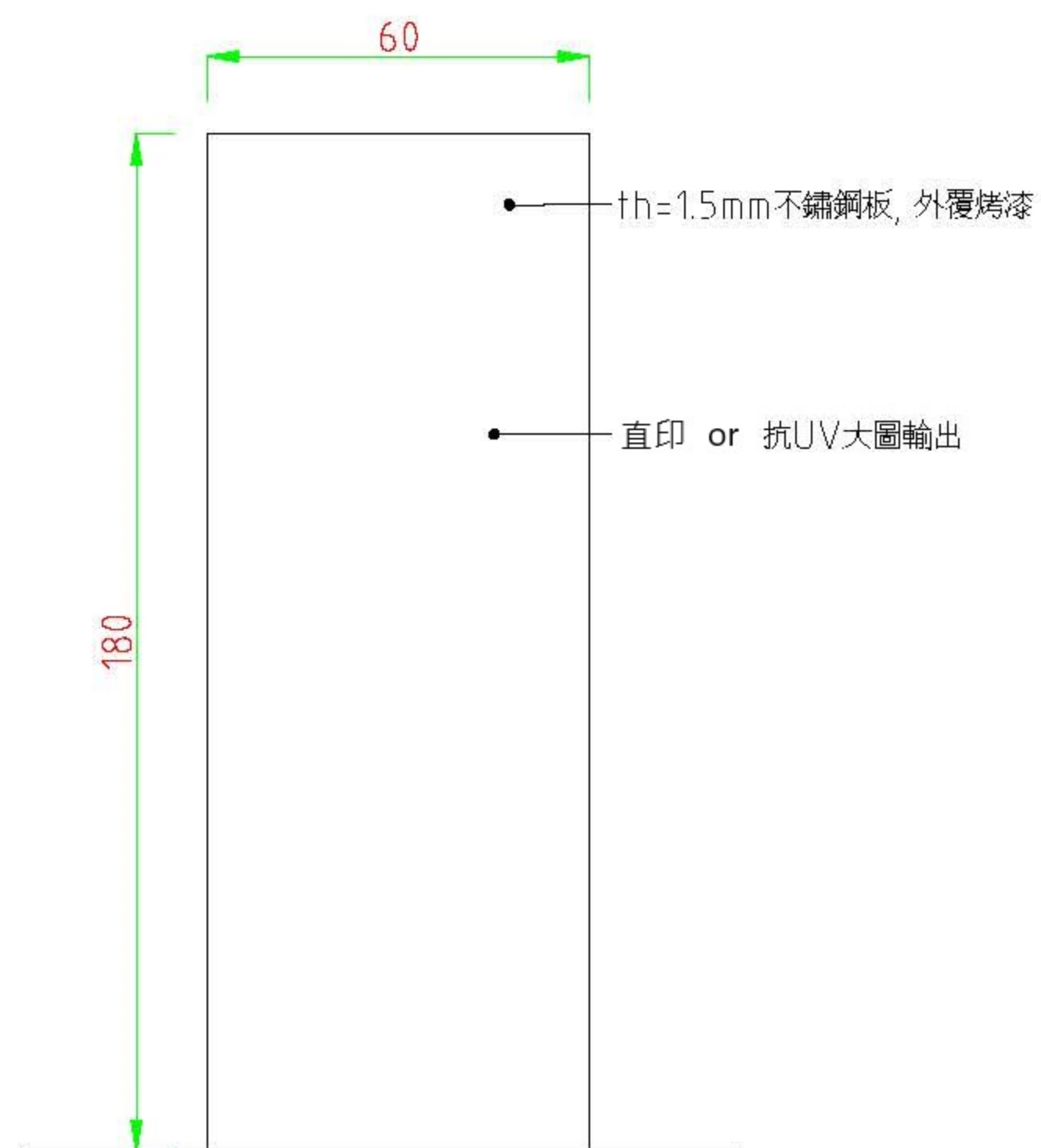
公園導覽牌正視圖
