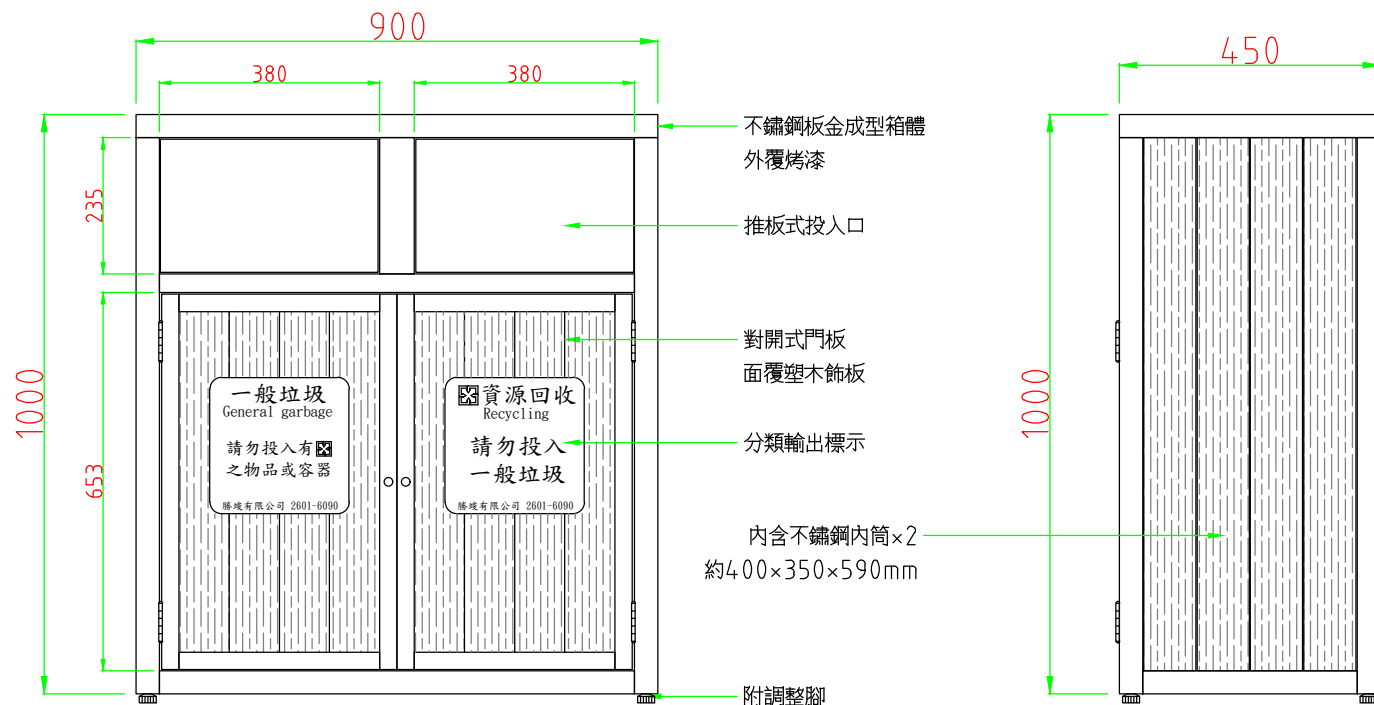
正視圖
