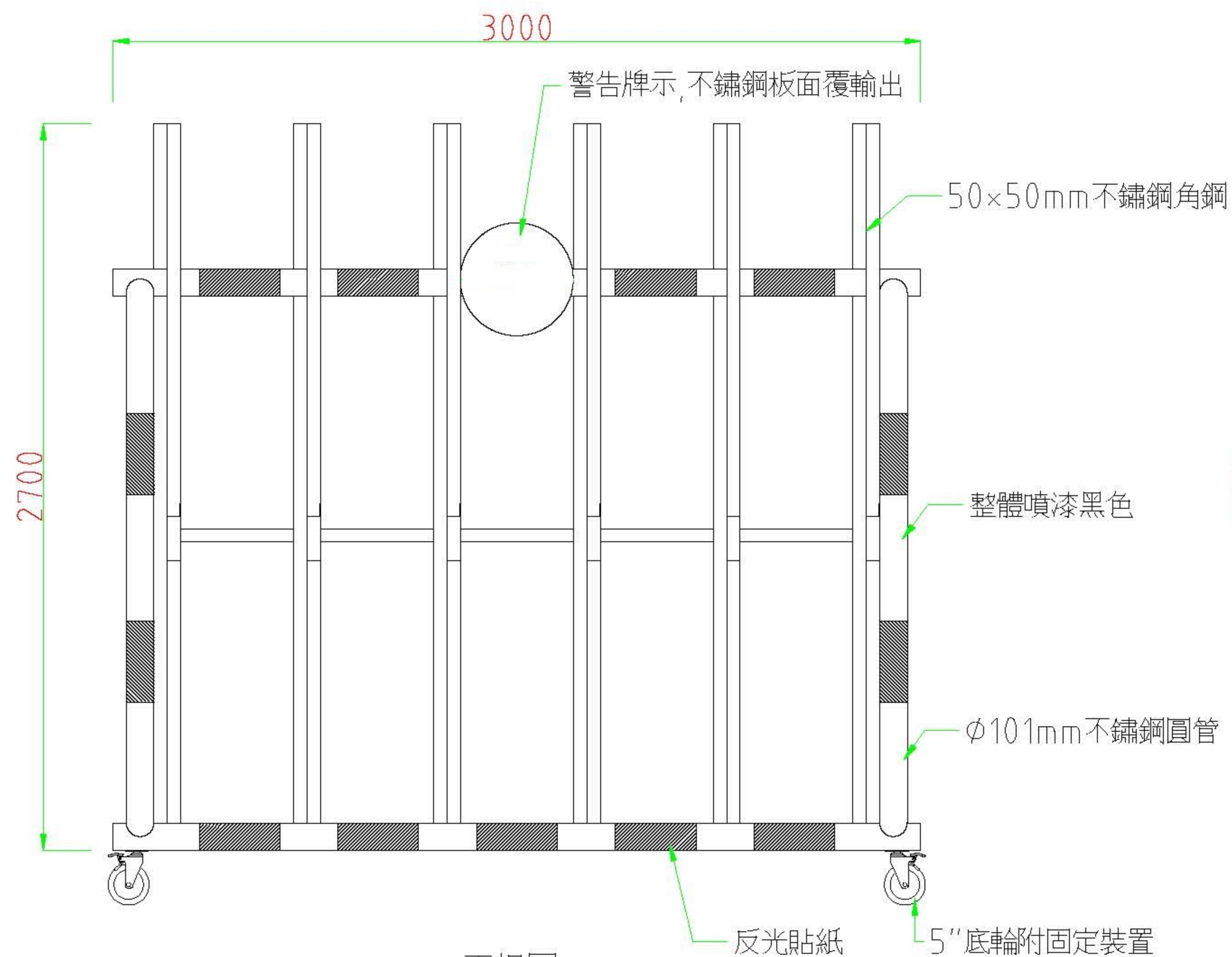
正視圖
