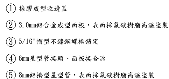
面板接合詳圖
