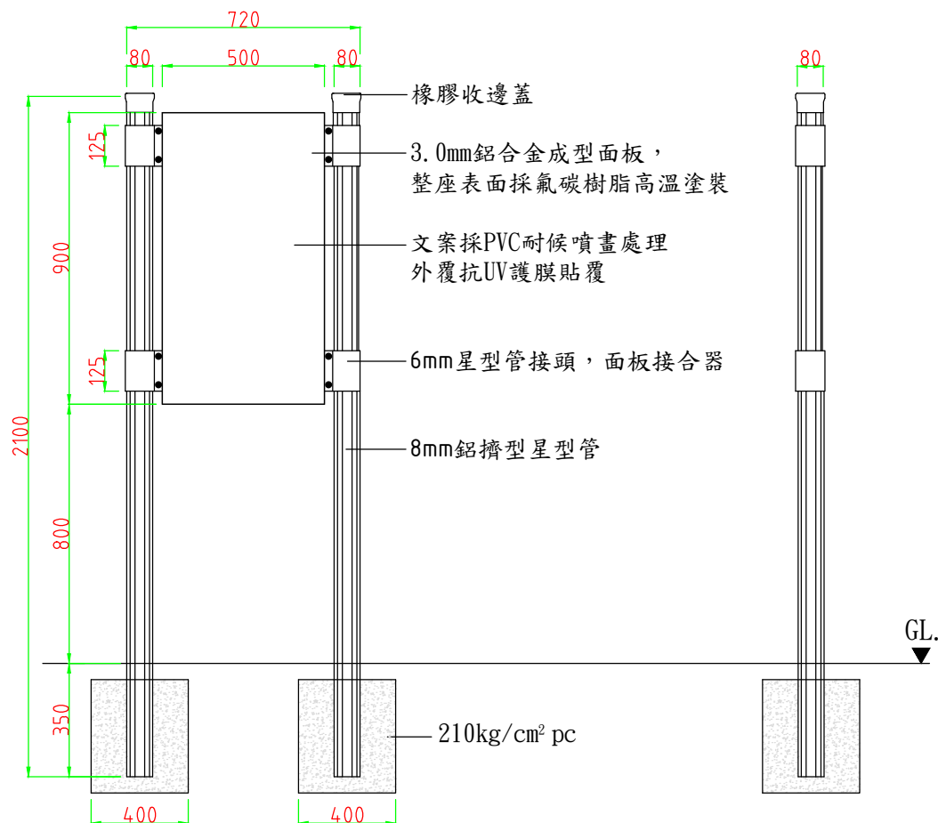
側視圖
