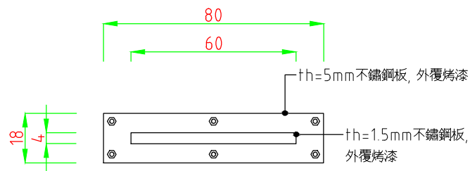
公園導覽牌上視圖
