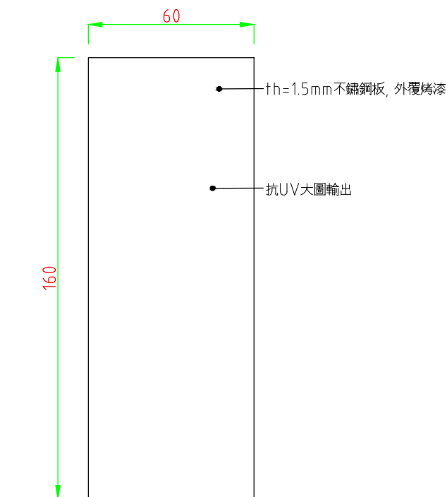
公園導覽牌正視圖
