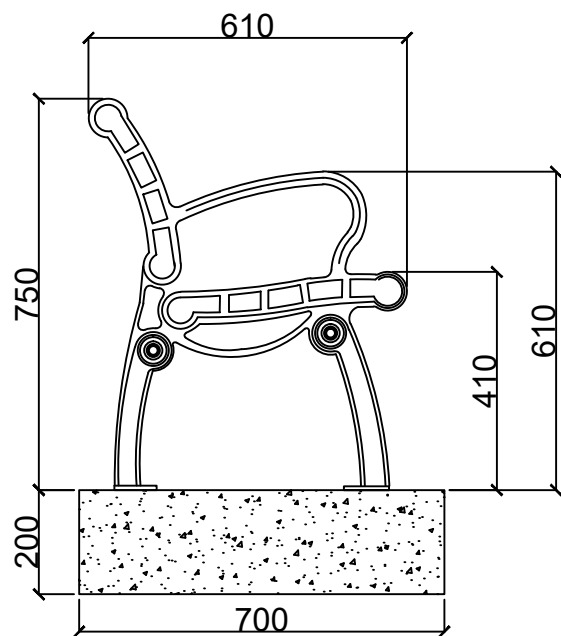
側立面圖
