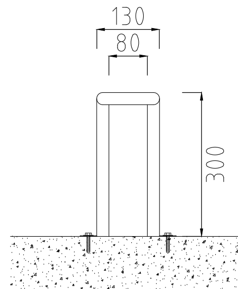
側立面圖
